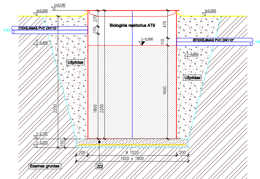
Pjūvis A-A'
